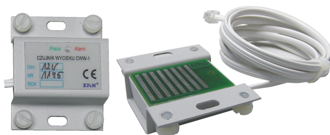
Rys.1 Widok czujnika wycieku wody CWW-1.
